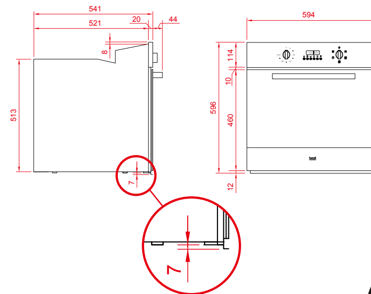
OV-367/OV-365*(OV-351)線圖
