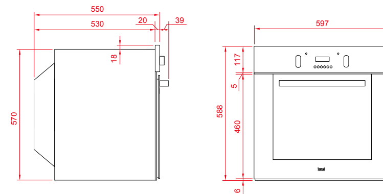
OV-367/OV-365*(OV-351)線圖
