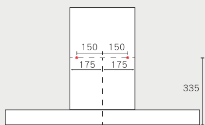
G-3110、G-3111 鎖點
